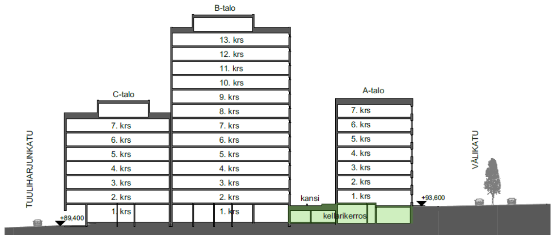
Kuva. Leikkauskuva kaavan viitesuunnitelman asuinkerrostaloista ja pysäköintihallista. Tuuliharjunkadun ja Välikadun välinen tasoero on yhden kerroksen verran. Tontin laajuinen Tuuliharjunkadun tasossa oleva pysäköintihalli tulkitaan maanpäälliseksi kerrokseksi. Välikatuun rajautuvan rakennuksen pysäköintihallin tasolla oleva kerros on kuitenkin maanalainen.
